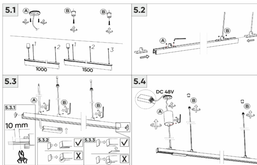
Sheme 5.1 5.4: baze i ovjesi, umetanje elemenata u utor, spajanje napajanja (48 V DC) i pode avanje.
