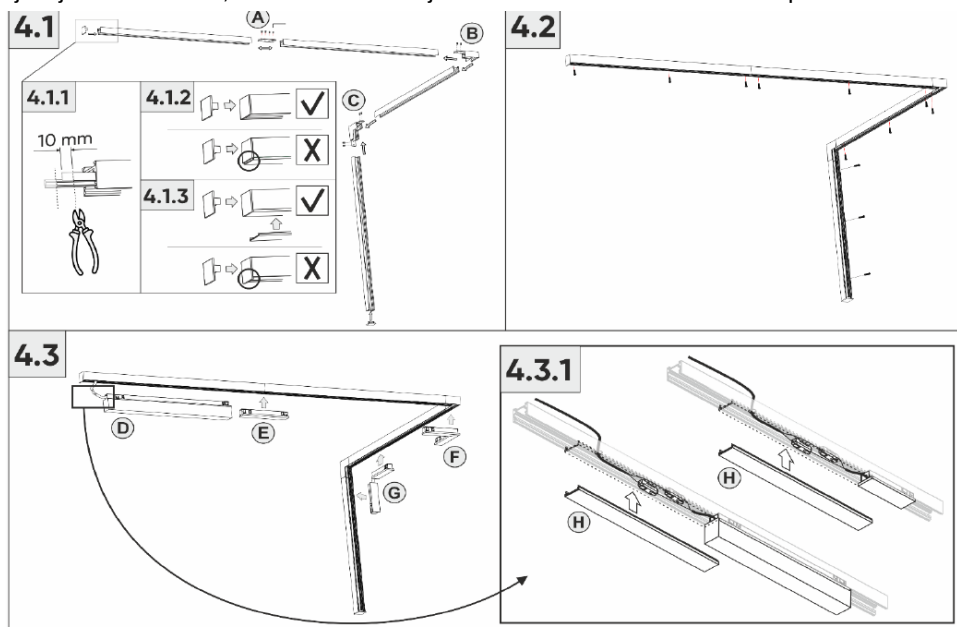
Sheme 4.1 4.3.1: sastavljanje, skraćivanje kontaktne grupe, monta a i ugradnja napojnog elementa i pokrova.
